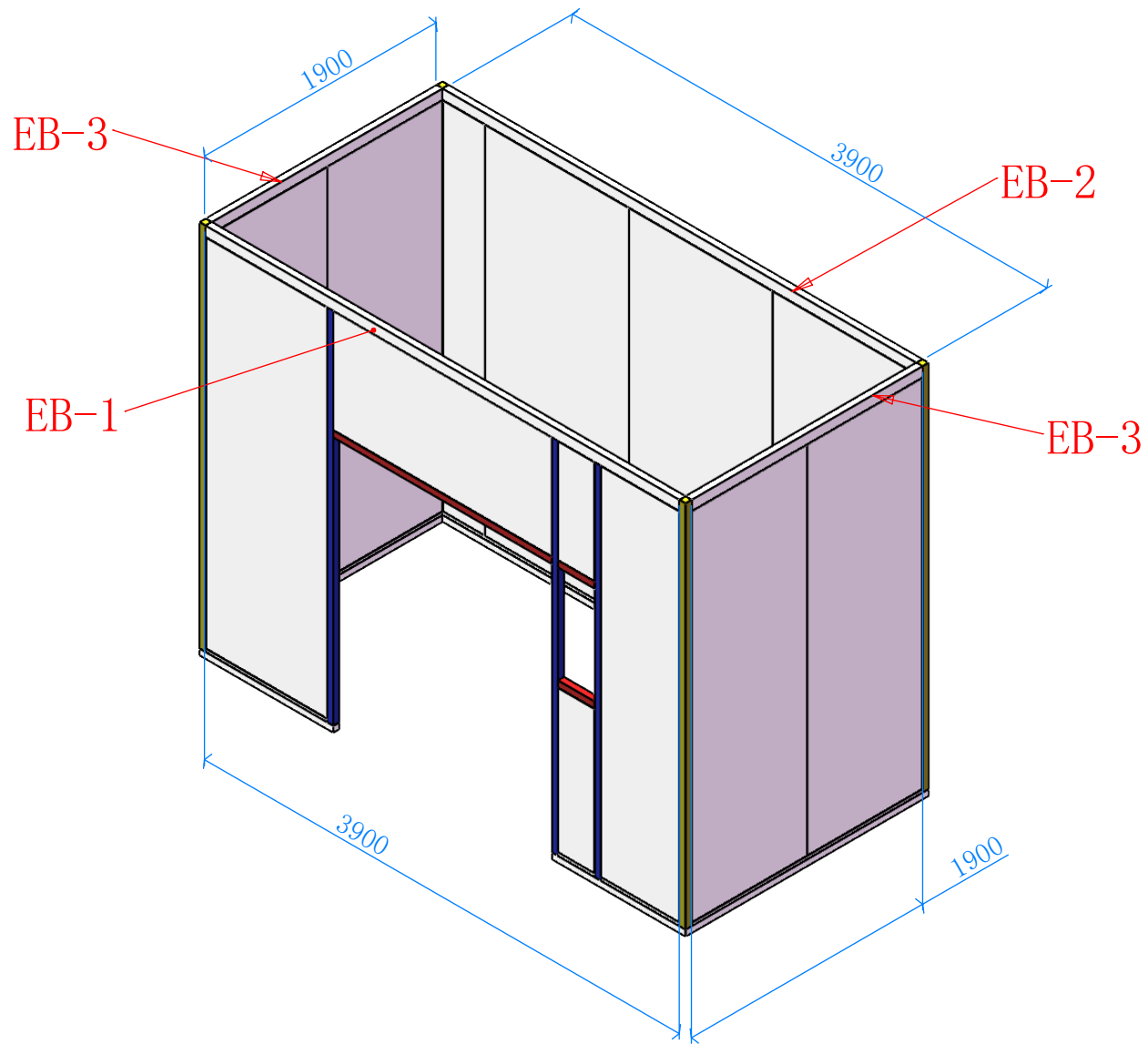
EDGE BEAM ASSEMBLY
